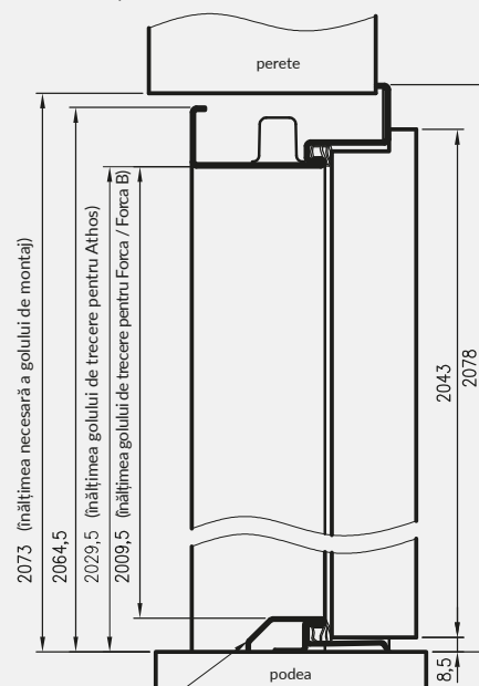
secțiune transversală verticală
