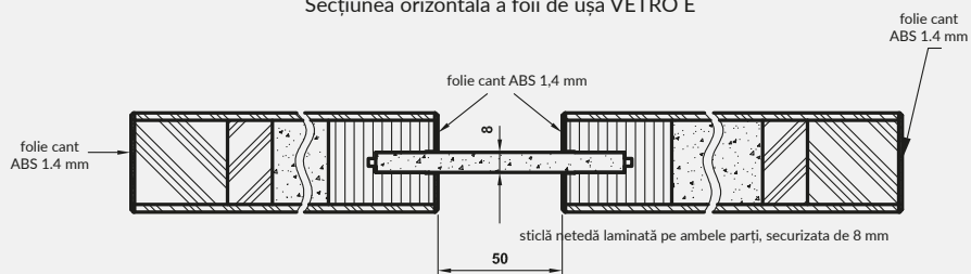
Secțiunea orizontală a foii de ușă VETRO E
