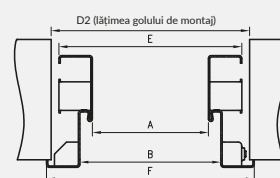
montaj secțiune transversală utilizând vată minerală
