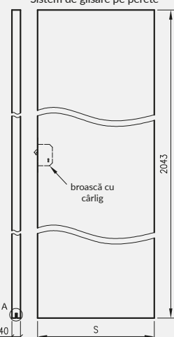
Uși glisante pentru: PA caseta Sistem SPAZIO CD Sistem de glisare pe perete
