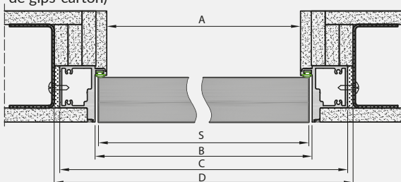
Sara Eco secțiune transversală orizontală (asamblare în perete de gips-carton)
