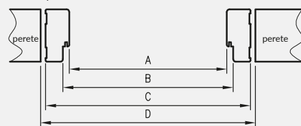
Sețiunea orizontală a tocului fix
