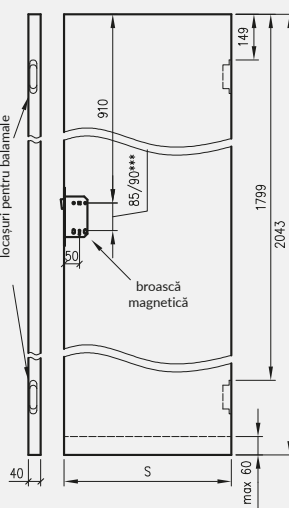
Ușă fără falt Sara Eco
