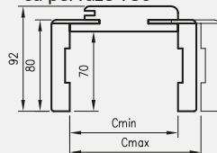
OR secțiune transversală cu pervaze T80
