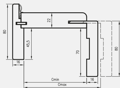
ORO secțiune transversală verticală
