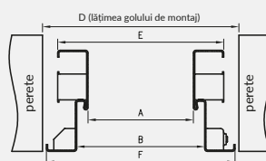
Dimensiuni pentru uși duble EI30
