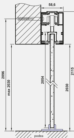
A - Secțiune transversală verticală Spazio TP
