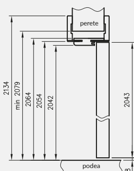
înălțimea necesară a golului de montaj 2079mm
