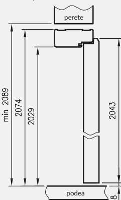
secțiune transversală verticală canat de ușă cu falț
