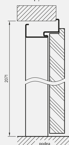
secțiune transversală verticală metoda opțională de asamblare
