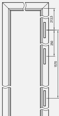
toc metalic pentru balamale VX 7939
