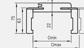
OR/ORC secțiune transversală cu pervaze T63
