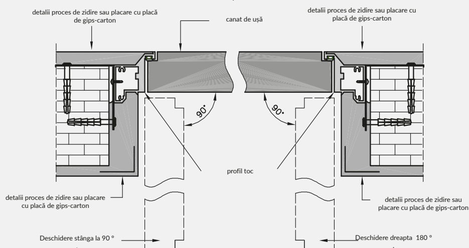
Sara Eco secțiune orizontală
