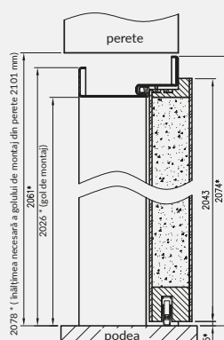
Secțiune verticală montaj utilizând vată minerală
