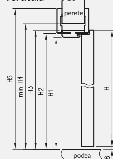
OR secțiune transversală verticală
