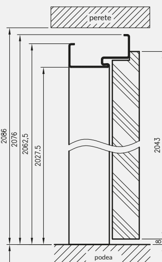
secțiune transversală metoda opțională de asamblare
