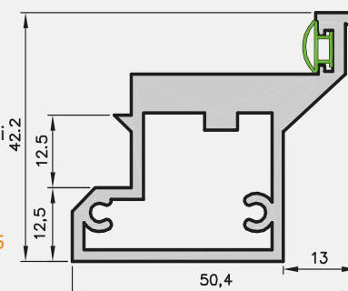
profil toc cu garnitură
