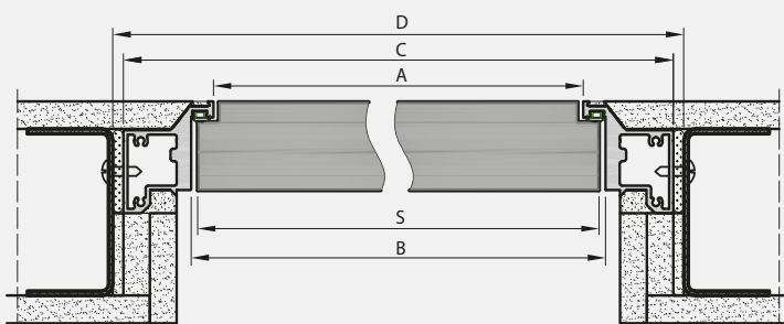
Dimensiuni ale foi de ușă Sara Eco
