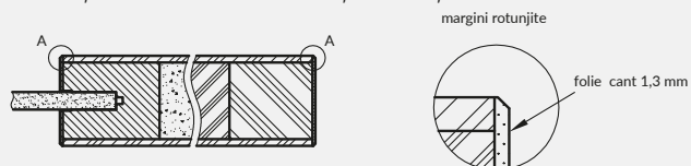
secțiune transversală a foi de ușă fără falț
