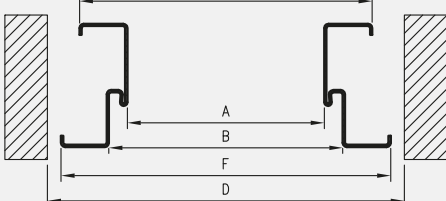
secțiune transversală
