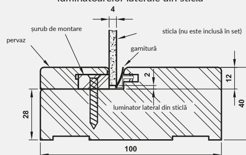
Fig. A Secțiune transversală supraluminilor și a luminatoarelor laterale din sticlă
