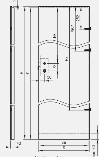
ușă fără falt Standard 10, Modern, Plus
