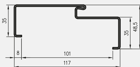
profil toc
