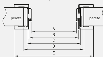
ORB secțiune orizontală
