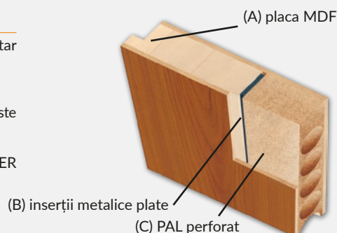
secțiune transversală ENTER natura
