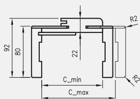
ORB secțiune transversală 075
