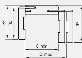
secțiune transversală TUN cu T63
