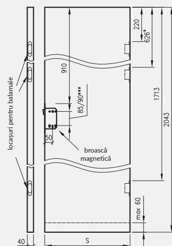
ușă fără falt
