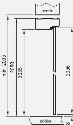
secțiune transversală verticală uși din sticlă
