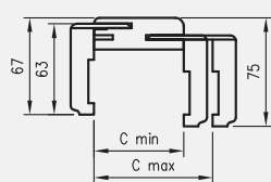
secțiune transversală TUN Natura cu N63
