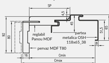
profil toc
