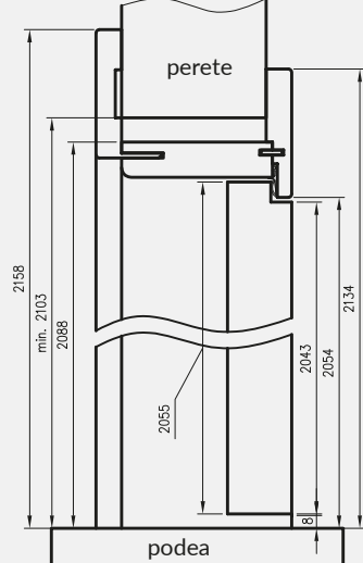
ORO secțiune transversală verticală
