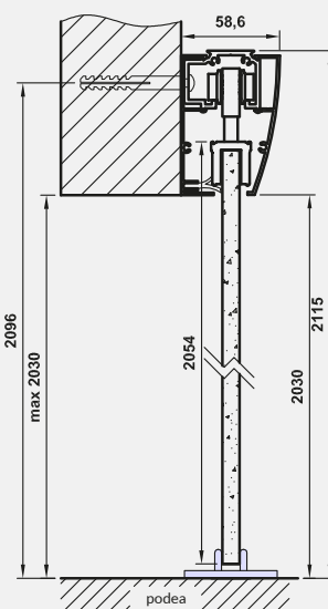
A - Secțiune transversală verticală Spazio TO
