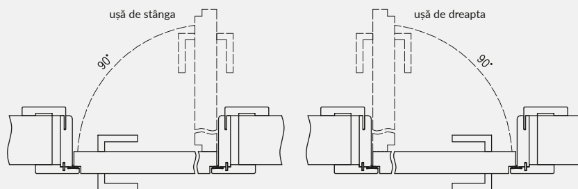
ORO secțiune orizontală
