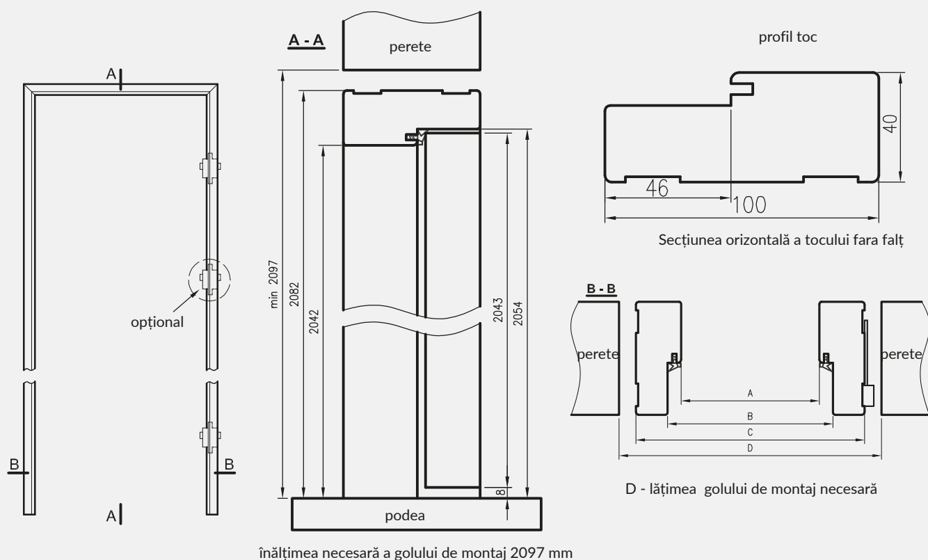
secțiune transversală verticală OPB canaturi de uși fără falț
