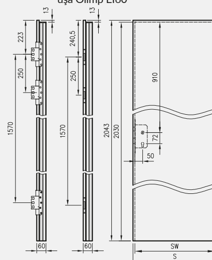
ușă Olimp EI60 **
