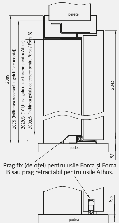
secțiune transversală toc reglabil metalic
