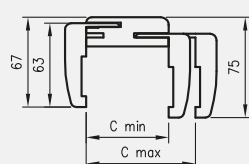
secțiune transversală TUN cu T80
