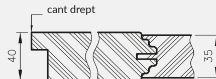
Secțiunea orizontală Nestor, Lexa
