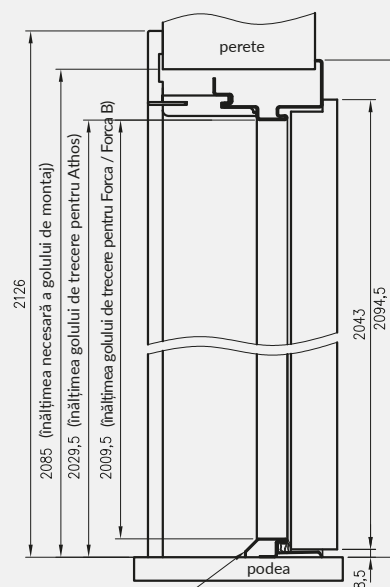
secțiune transversală verticală
