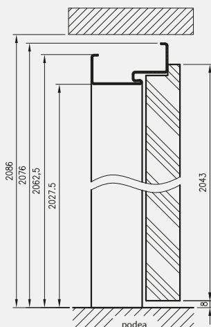
secțiune transversală metoda opțională de asamblare
