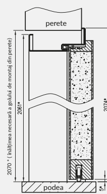
Secțiune verticală montaj utilizând beton
