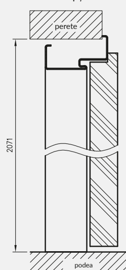
secțiune transversală verticală metoda opțională de asamblare
