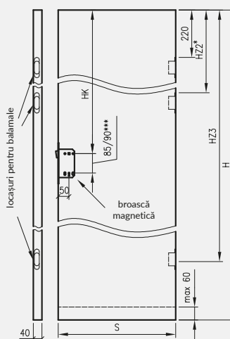
ușă fără falt Standard 10, Modern, Plus
