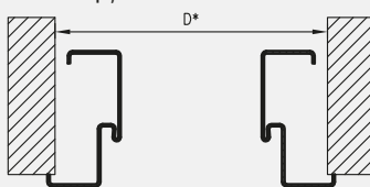
secțiune transversală metoda opțională de asamblare
