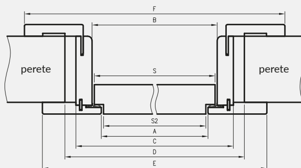
ORO secțiune orizontală
