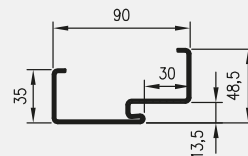
secțiune transversală toc metalic
